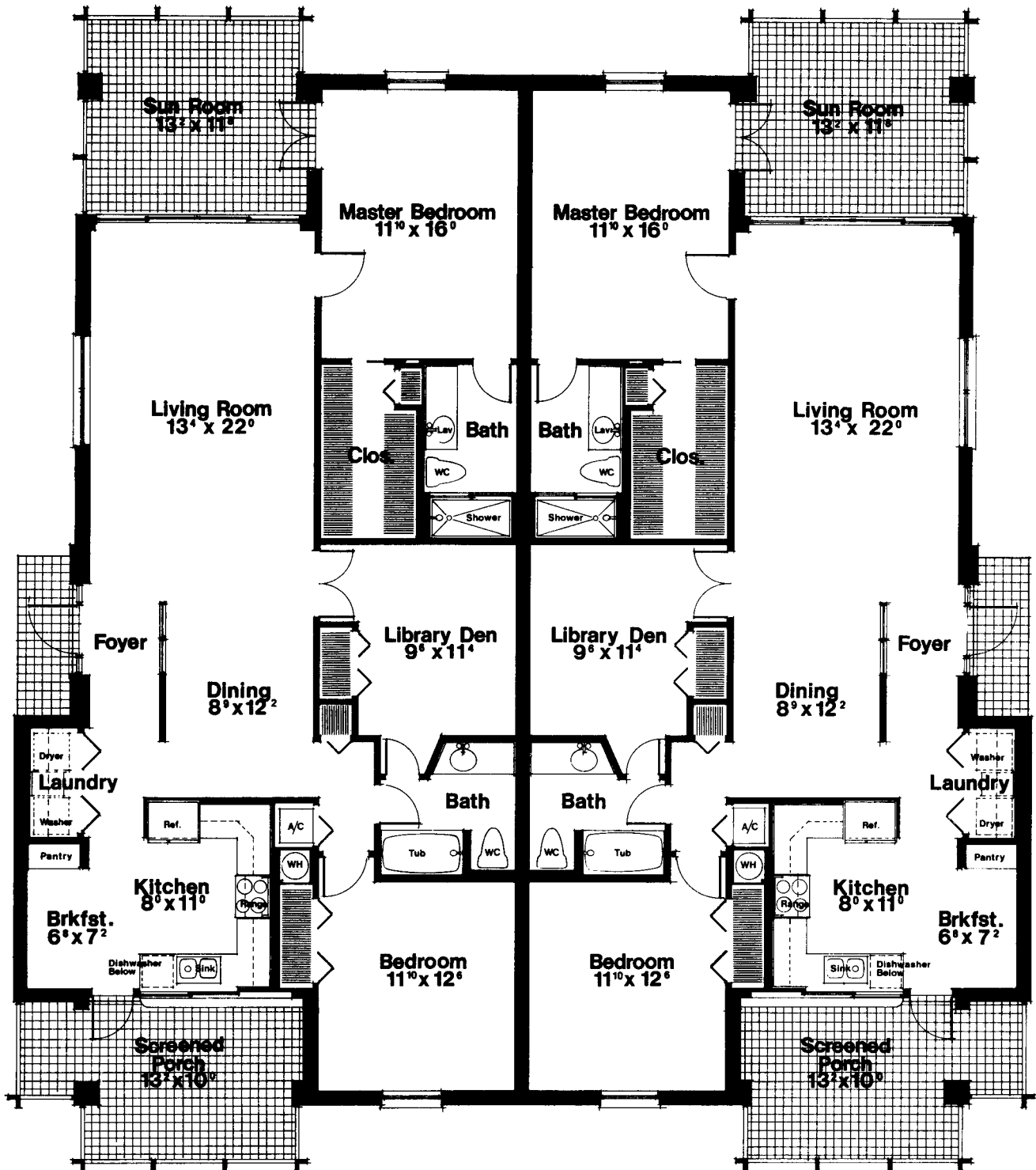
T y p i c a l A p a r t m e n t P l a n
